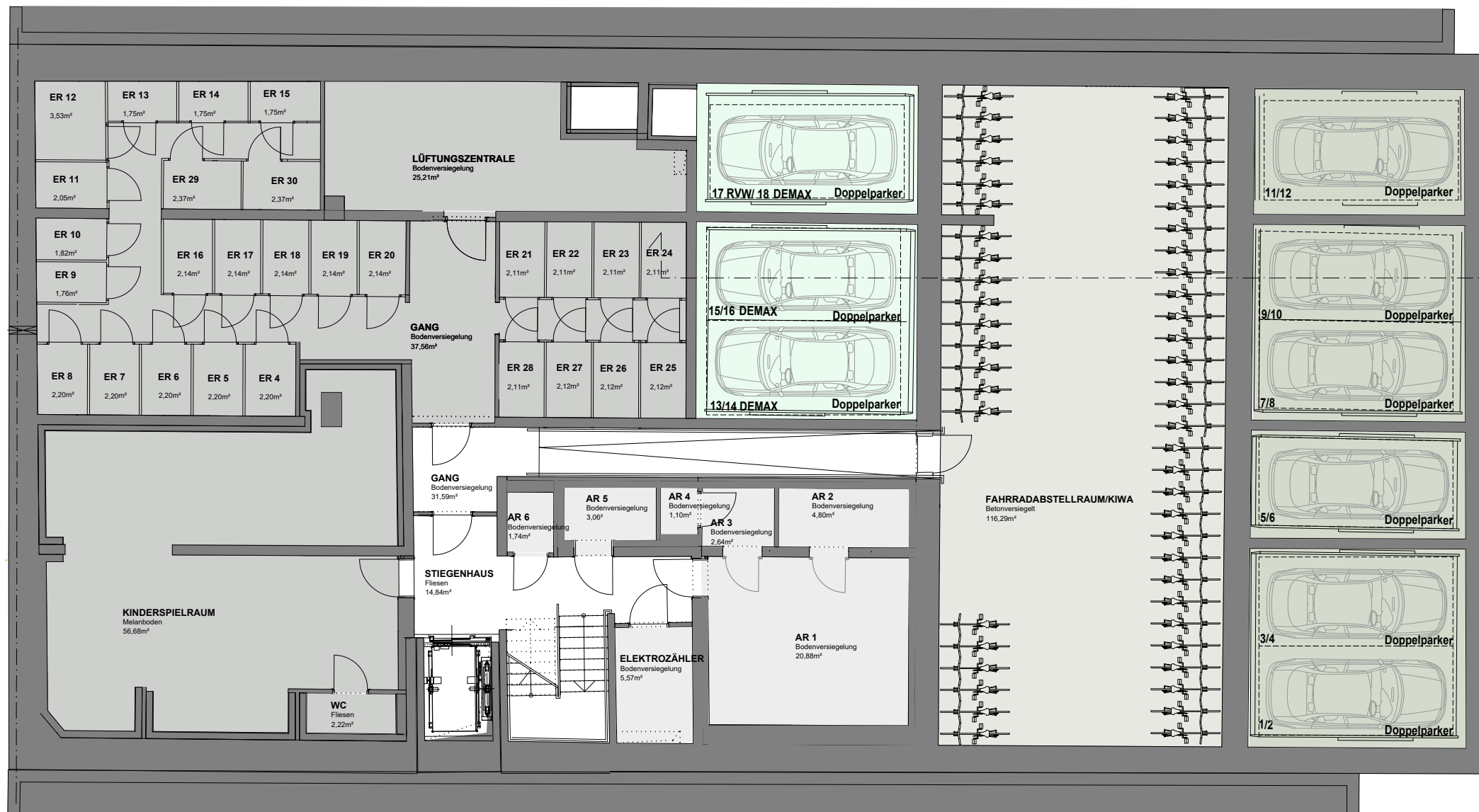
A 2. KELLERGESCHOSS
